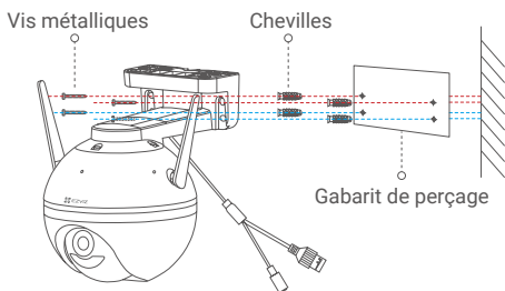
Fig. 1 Montage mural
